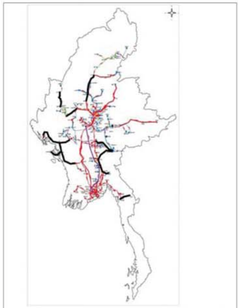
ဝန်ပိုများ ထမ်းဆောင်နေရသည့် လက်ရှိအသုံးပြုနေသည့် ဓာတ်အားလိုင်းများ ဖျက်ဆီးခံထားရသည့် ဓာတ်အားလိုင်းများ (၂၆-၁၇ %)
